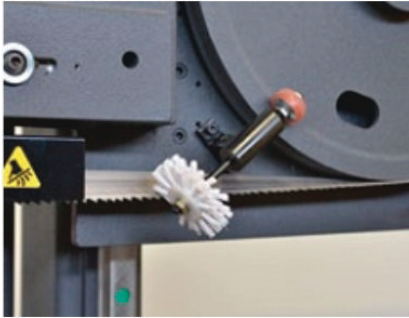
Savbåndsbørste
