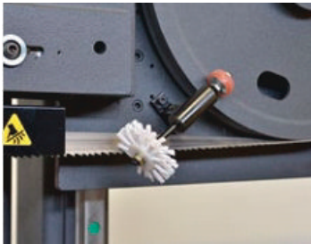
Savbåndsborste
