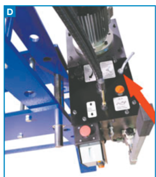
2 pressehastigheder. Trin 1 presser 2,3 m/pr. sek. Trin 2 presser 9,5 m/pr. sek.
